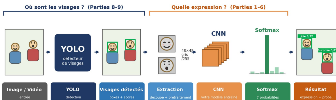
Figure 4 — Pipeline complet du projet : Image/Vidéo → YOLO → visages détectés → extraction → CNN → Softmax → expression + probabilité.
