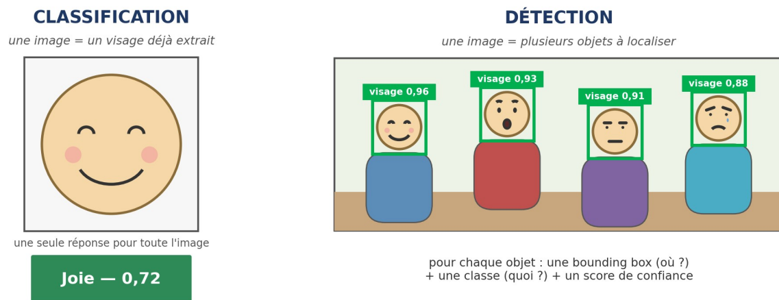
Figure 3 — Classification vs détection : à gauche, une seule réponse pour l'image ; à droite, une bounding box et un score pour chaque visage.
