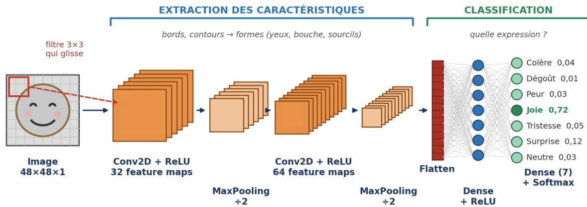
Figure 2 — Principe d'un CNN appliqué à la reconnaissance d'expressions (exemple d'architecture, à adapter).
